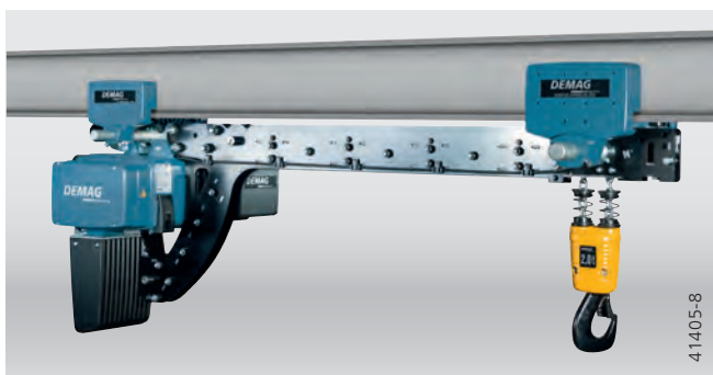
Chariot court avec course de crochet augmentée
