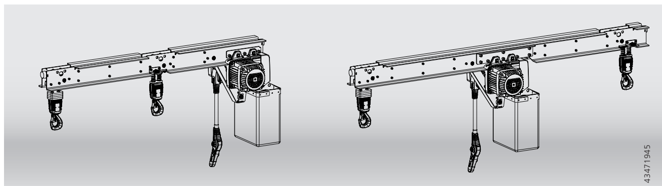
Palan à double sortie de chaîne KLDC-D : encombrement vertical réduit, positions de sortie 3/4 et 4/5
